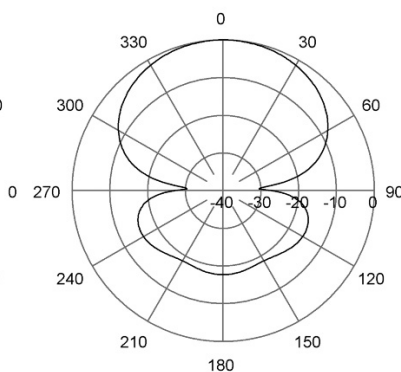
H-Plane | 445 MHz
