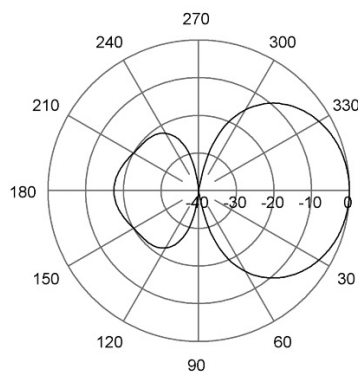
E-Plane | 445 MHz
