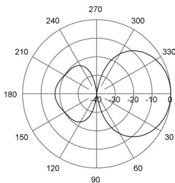
E-Plane | 400 MHz
